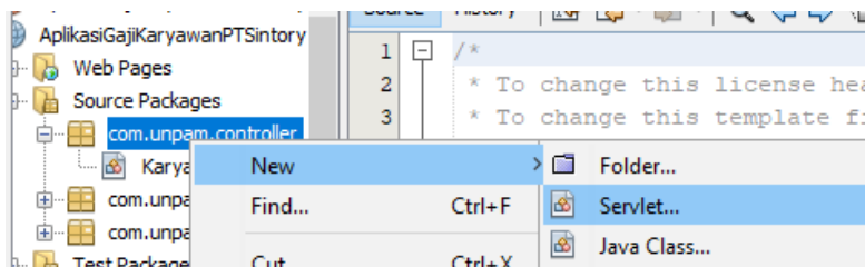
Gambar 249. Membuat Servlet
