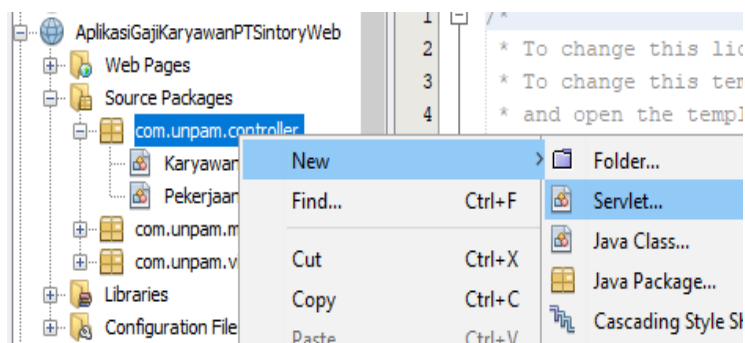
Gambar 254. Membuat Servlet
