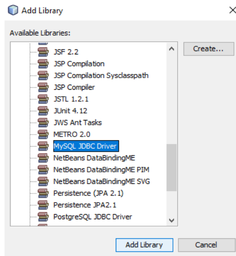
Gambar 265. Memilih Library
