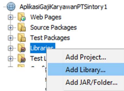
Gambar 264. Memilih Library
