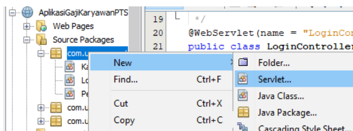
Gambar 259. Membuat Servlet
