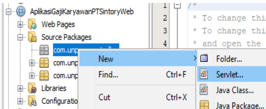
Gambar 244. Membuat Servlet
